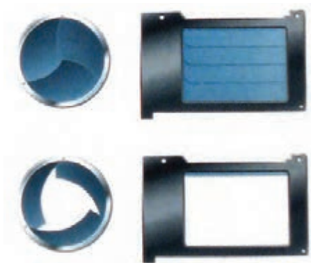
تصویر ۲-۲- شاترهای مرکزی و کانونی در ۲ حالت باز و بسته
