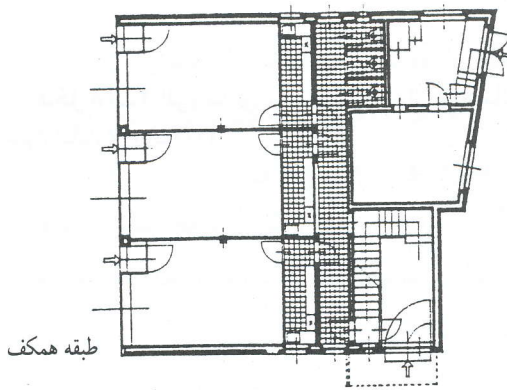
شکل ۳۷-۳ آلبرتو سارتوریس، مجتمع آپارتمانی و خدماتی، جنوا، ایتالیا، ۱۹۳۶-۱۹۳۷. در طبقه همکف این مجتمع سه فروشگاه، دفاتر کوچک و سرویسها قرار دارند. طبقات اول و دوم شامل: آپارتمان و تراس روبه جنوب و طبقه سوم شامل یک سوئیت و تراس آفتابگیر است.
