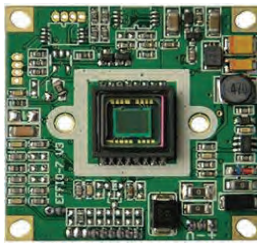
تصویر ۲۳ جانمایی واقعی CCD
