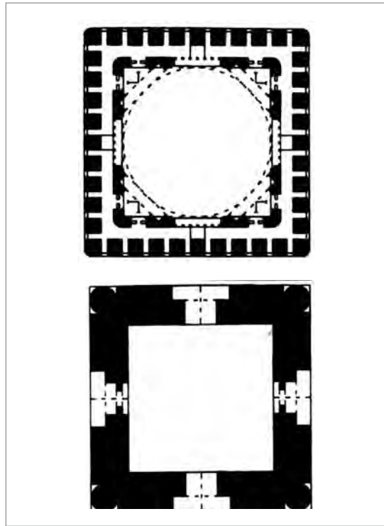
شکل ۱-۱۵۵- پلان مقبره امیراسماعيل سامانى در دو ارتفاع شکل ۱-۱۵۶- تصویر سه بعدی خارجی مقبره امیراسماعيل سامانى
