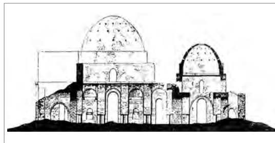
شکل ۱-۱۴۰- برش از اتاق گنبددار کوچک
