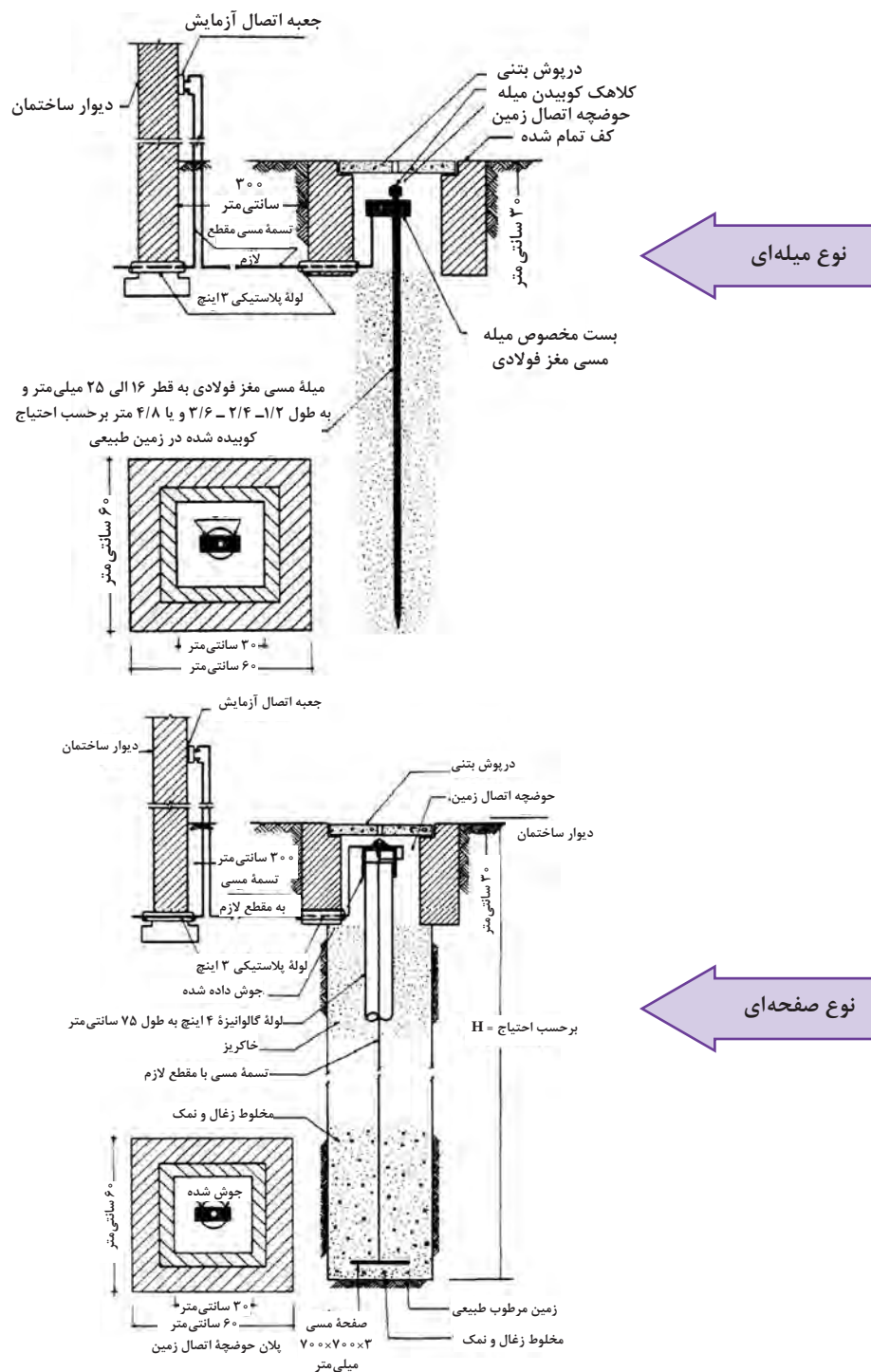
شکل ۳-۱۳- جزئیات (دتایل) اجرایی سیستم اتصال زمین با چاه ارت و میله
