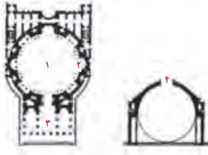
۱ گنبدخانه ۲ تاقچه (جایکره دیواری) ۳ رواق ورودی ۴ نورگیر گنبد
