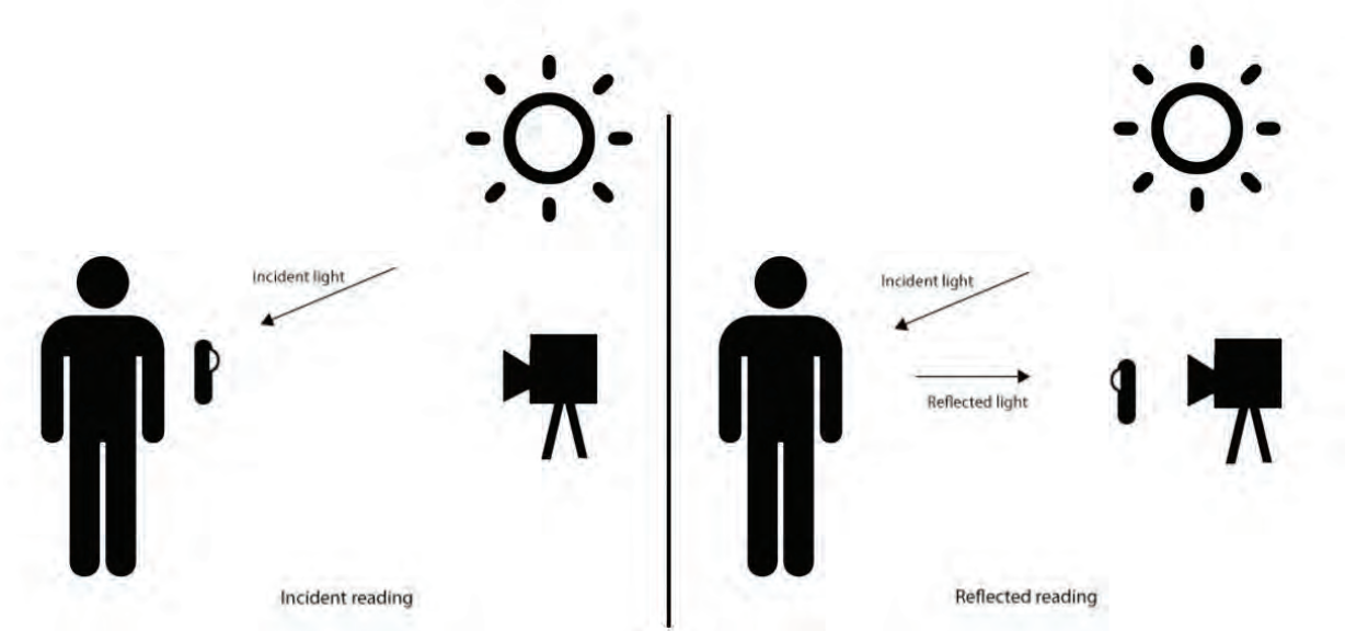
▲ تصویر ۱۹۷ | نورسنجی مستقیم
