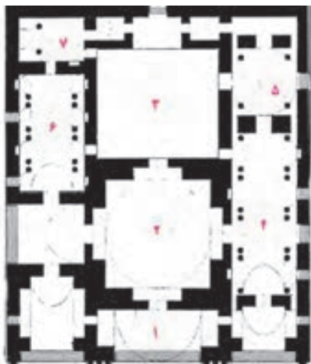
تصویر شماره ۳۰-۲- نقشه کاخ سروستان
