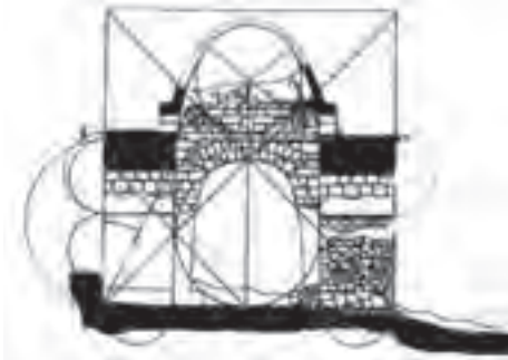
تصویر شماره ۵-۳- مقطع و نقشه آتشکده
