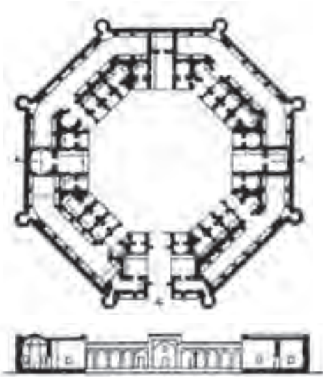
تصویر شماره ۱-۴- کاروانسرای خان خوره، جاده شیراز به آباده مربوط به دوره صفوی
