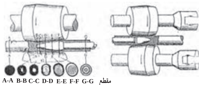
شکل ۵-۱۰- تولید لوله بدون درز توسط مغزی گذاری
