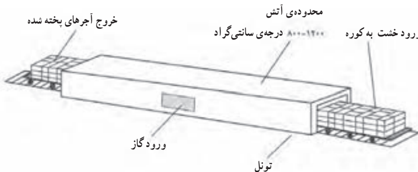
شکل ۶-۷- کوره‌ی تونلی
