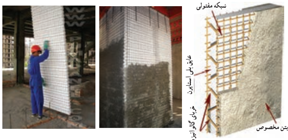
شکل ۱۵-۳ جزئیات دیوار سبک و نحوه ی اجرای آن
