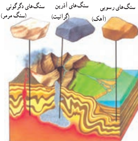
شکل ۳-۴ نحوه‌ی تشکیل انواع سنگ‌ها
